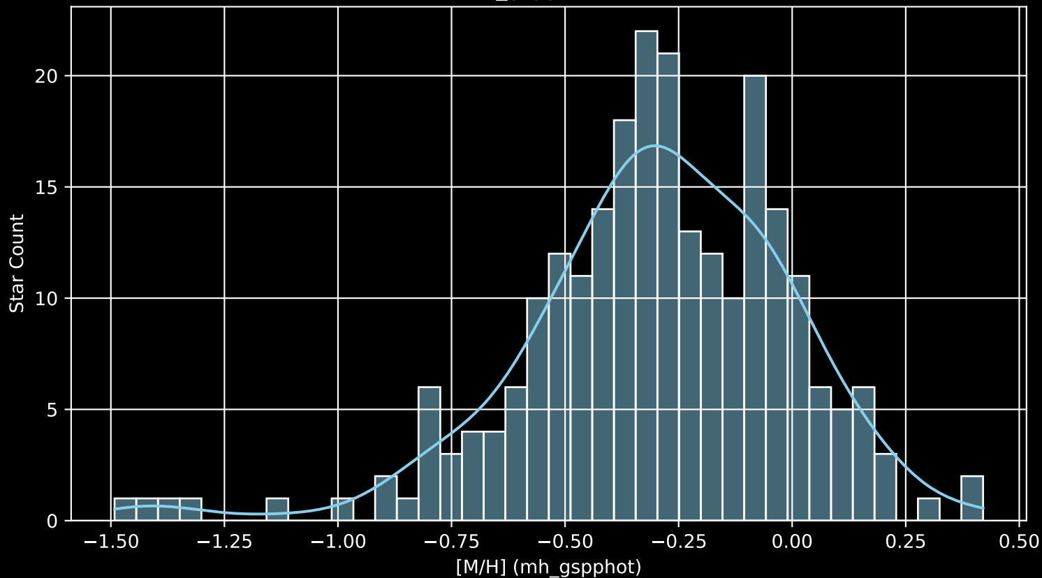
GALAH DR4 Field: [7131] [M/H] (mh_gspphot) (n= 243)
