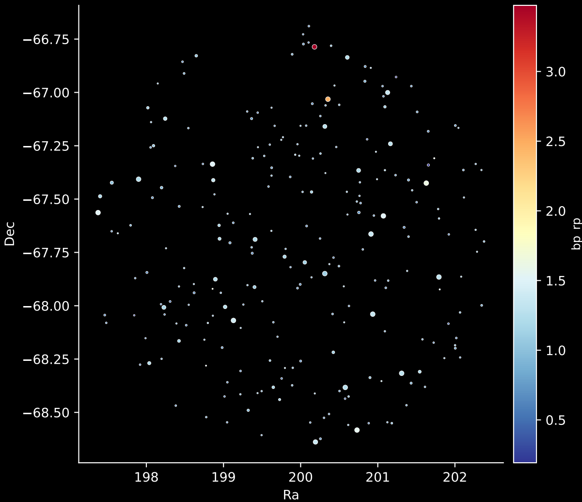
GALAH DR4 Field: [7131] Stars: 243
