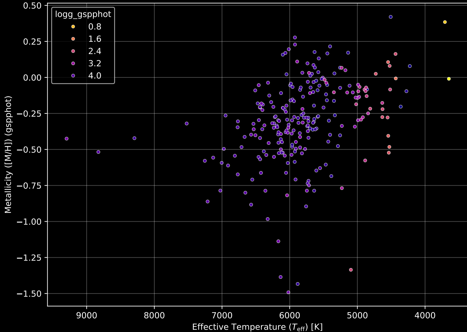
GALAH DR4 Field: [7131] Stellar Population Parameters (n= 243)
