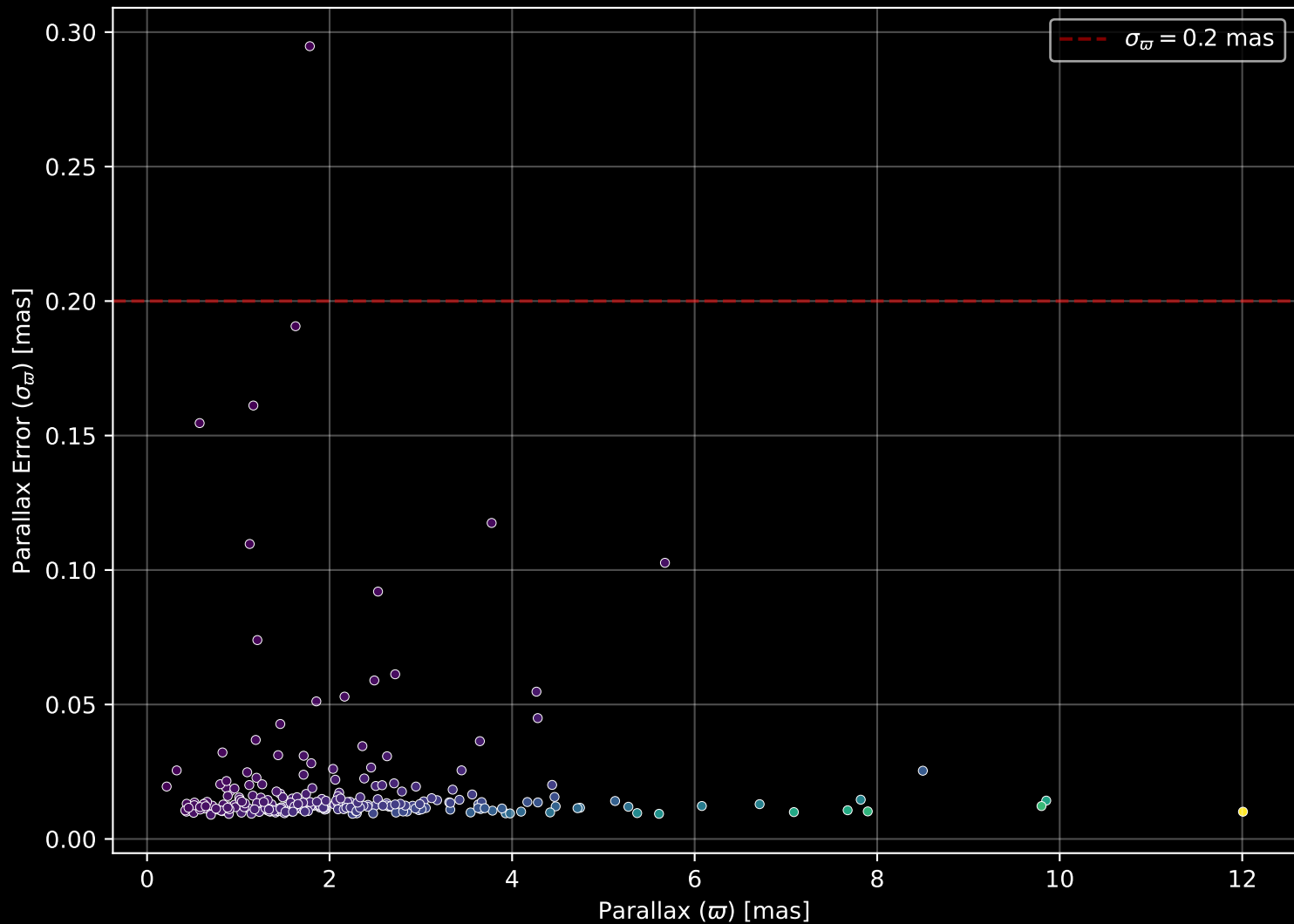
GALAH DR4 Field: [7131] Parallax Quality (n= 243)
